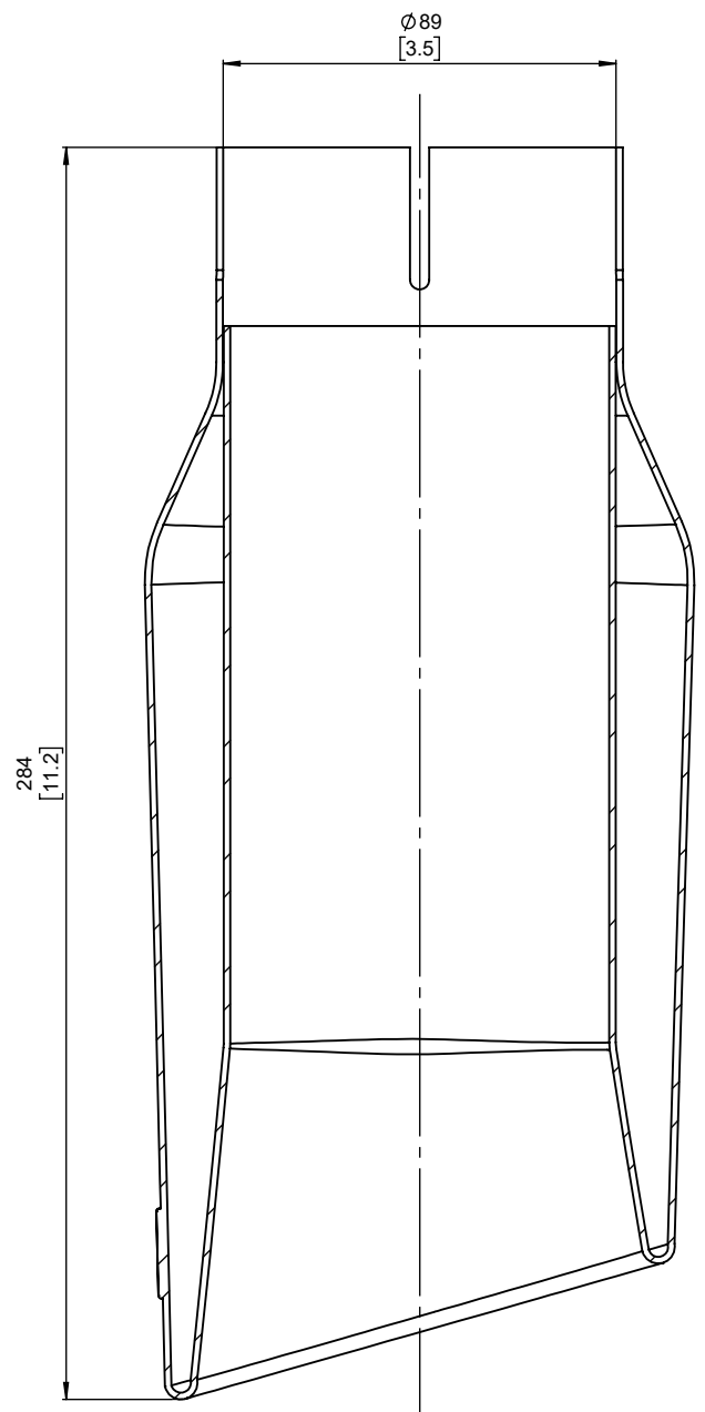
SECTION A-A
