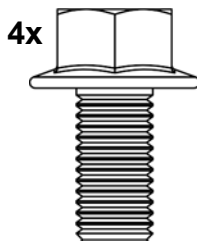
M10-1.25 x 20mm Lg. FHCS
